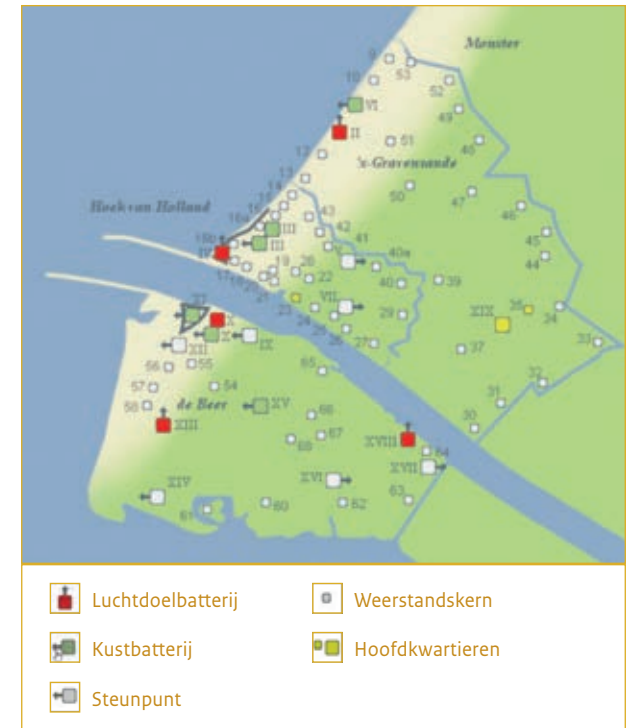
Overzicht van de bouwwerken van de Festung Hoek van Holland. Bron: Atlantikwall-museum.
