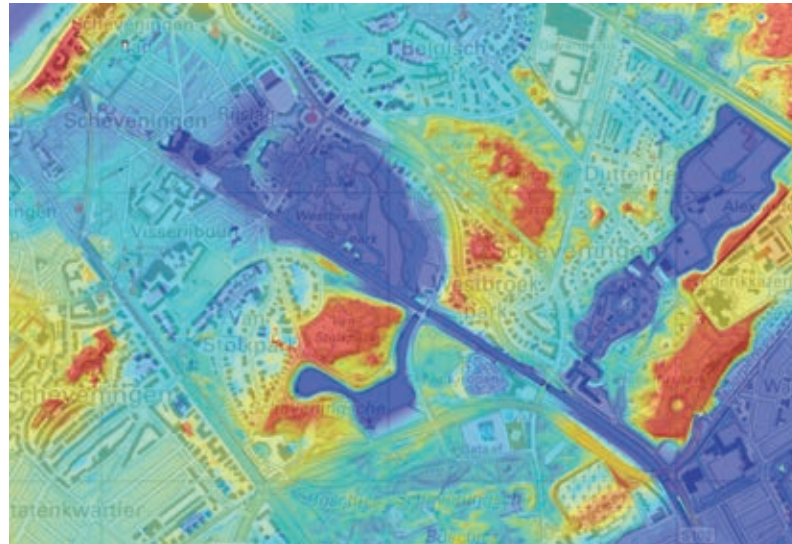
Hoogtebeeld (AHN2) van het in de jonge duinen gebouwde deel van Den Haag en Scheveningen. In de Scheveningse Bosjes is nog duidelijk het duinreliëf zichtbaar. In de Nieuwe Scheveningse Bosjes geldt dat zelfs voor de kop van een grote paraboolvormige duin. Zichtbaar is ook dat de Scheveningse Weg, geheel volgens de zeventiende-eeuwse principes, nauwkeurig is geëgaliseerd (zie deel 5 hoofdstuk 2). De laagtes van de Waterpartij, het Westbroekpark en Klein Zwitserland ontstonden door zandwinning.
